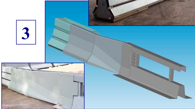
Raccordement profil SAFEGUARD sur profil VARIOGUARD
